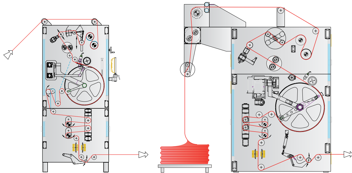
Kombi weftstraightener
